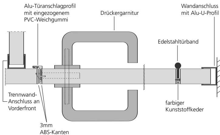
Zeichnung: Kabinenanlage Typ SVF30
