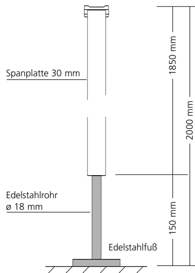
Zeichnung: Schnitt
