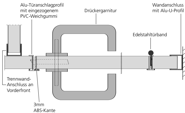
Zeichnung: Kabinenanlage Typ SV30
